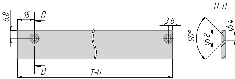
Планка торцевая (SK0125X3A), правая (левая, зеркальное отоб.)
