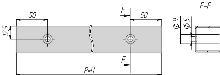
Угловой элемент (SK0125X25A)
