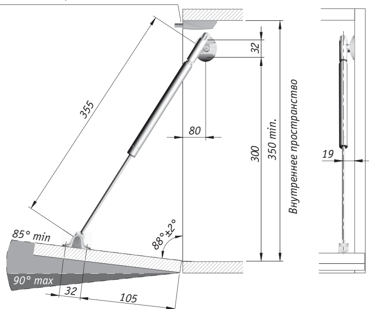
Толкатель K-PUSH TECH короткий с магнитом врезной или накладной
