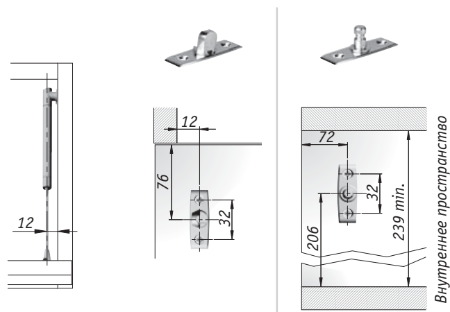
Использование креплений под саморез
