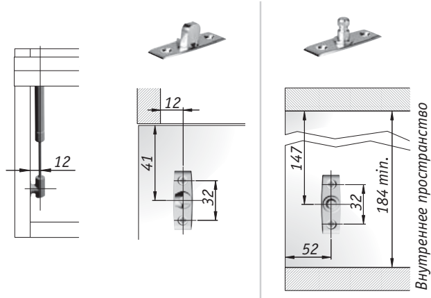
Использование креплений под саморез
